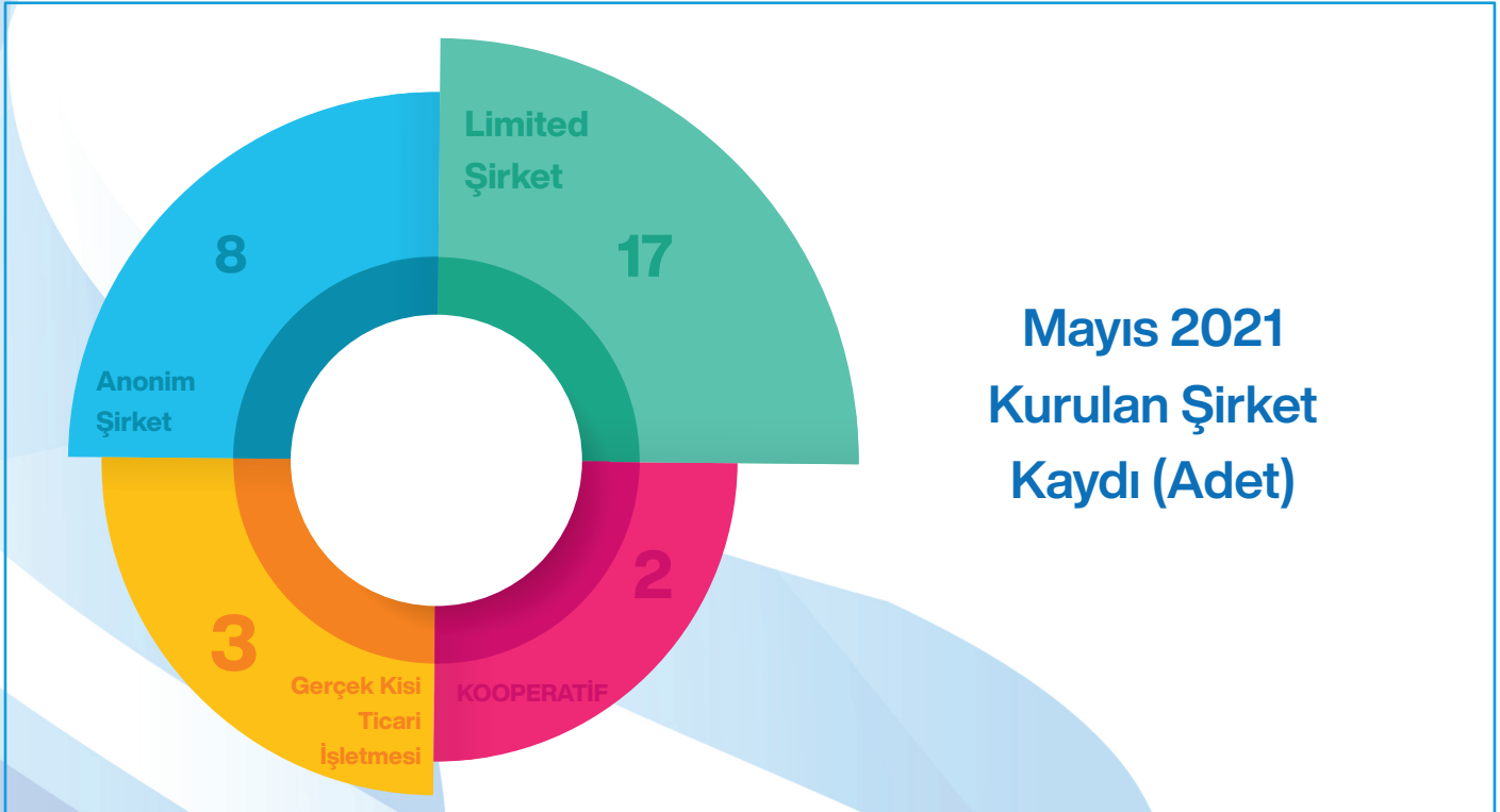
Grafik 11 - Sivas Ticaret ve Sanayi Odası Yeni Kayıt Üye Dağılımı
